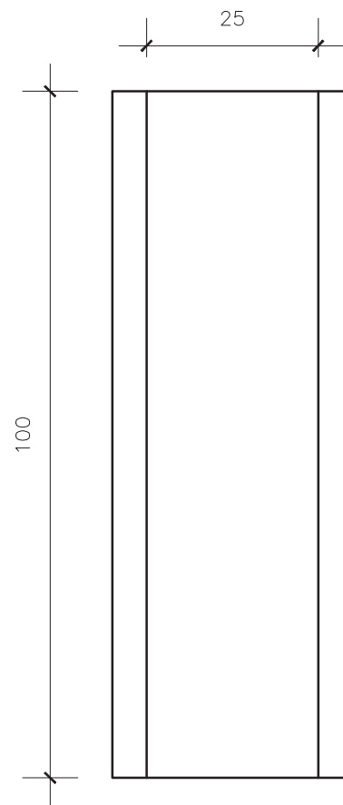
VISTA SUPERIOR
