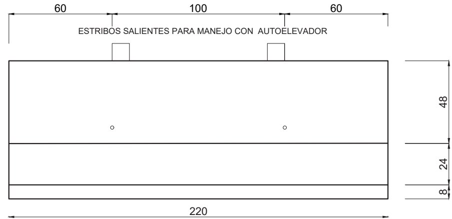
VISTA LATERAL ESC. 1:20
