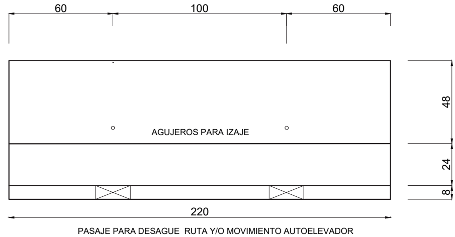
VISTA LATERAL ESC. 1:20
